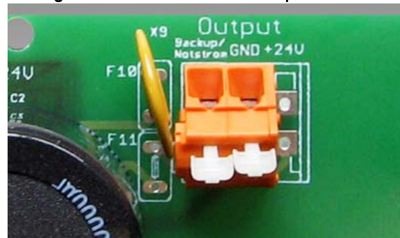
Abbildung 4: SHEV® 6 – Klemme Backup/Notstrom
