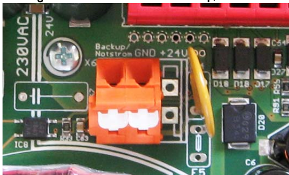
Abbildung 2: SHEV® 3 – Klemme Backup/Notstrom
